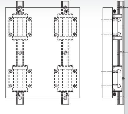
Vertical (Code : V)
